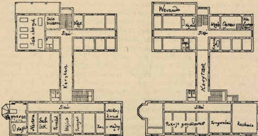
Szpital i przytułek dla kalek w Salzuflen. Piętro.
